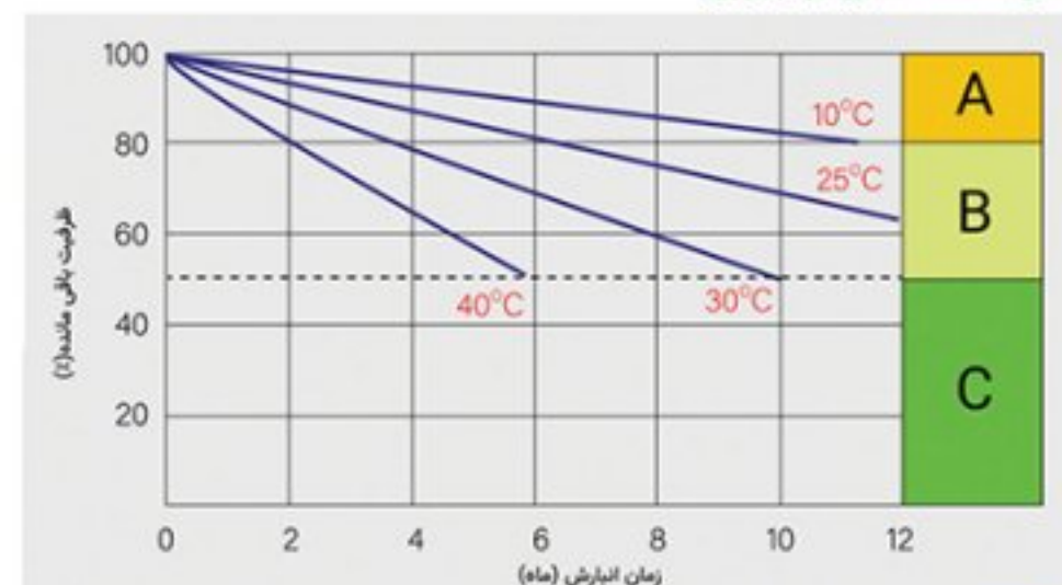
منحنی مشخصه دشارژ خود بخودی
