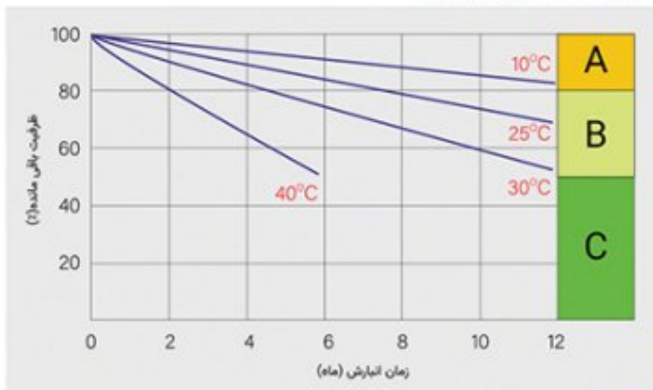
منحنی مشخصه دشارژ خود بخودی
