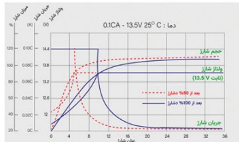
منحنی مشخصه شارژ شناور
