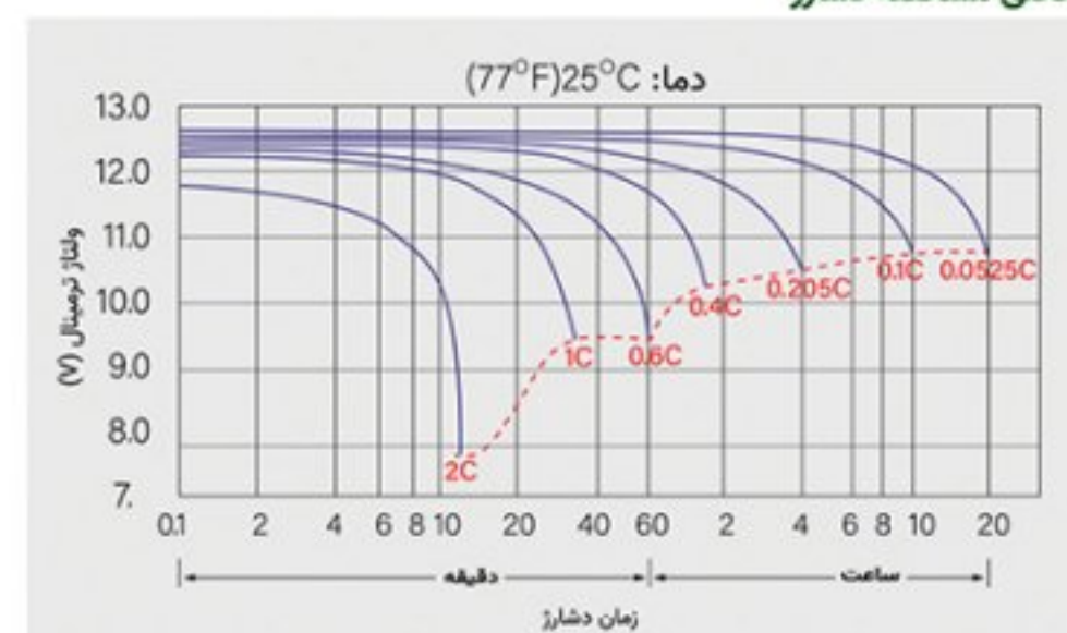
منحنی مشخصه دشارژ
