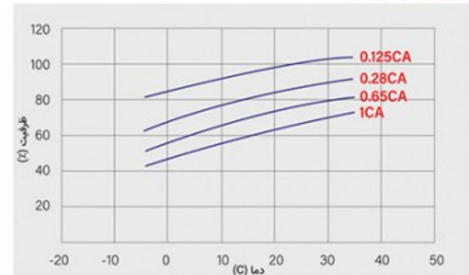
اثر دما نسبت به ظرفیت
