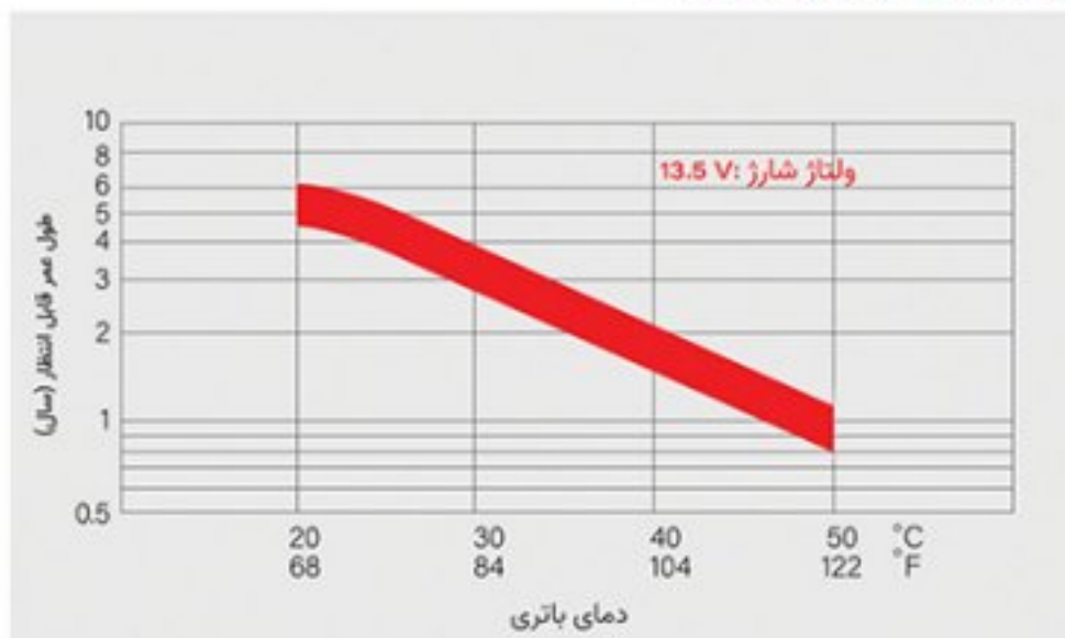
اثر دما بر عمر شناور در طولانی مدت
