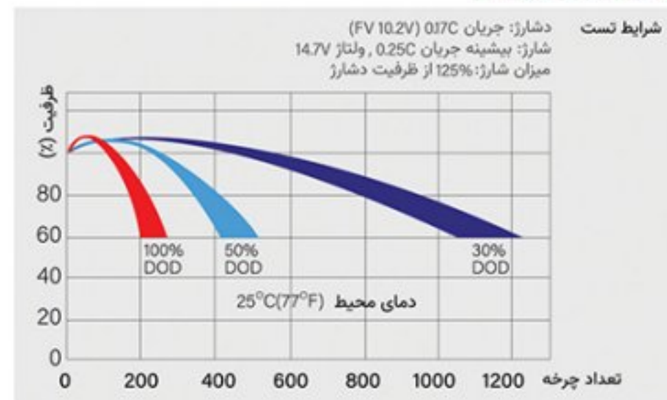
منحنی مشخصه شارژ
